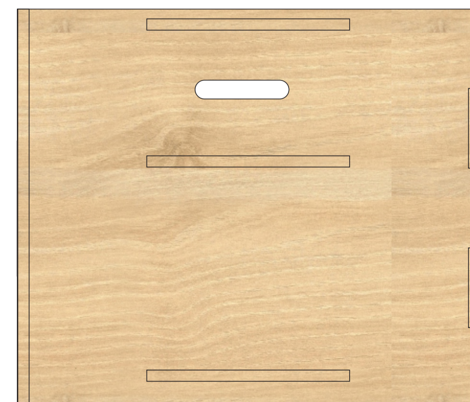
коробка_вид слева
