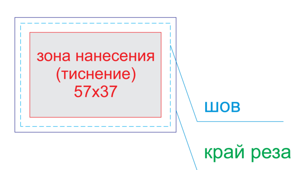
ПАТЧ ПРЯМОУГОЛЬНЫЙ
