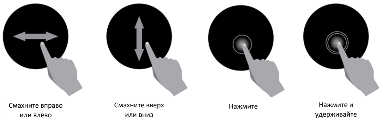
Рисунок 5 – Поддерживаемые жесты
