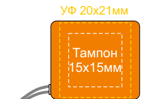
Вид сверху
